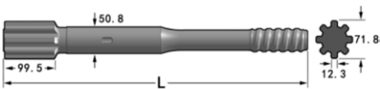
Furukawa HD 712
